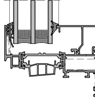
CAM KALINLIĞINA GÖRE CAM ÇİTASI SEÇİM TABLOSU KANAT-KANAT İÇİ ORTAKAYIT-ETEK PROFİLİ Glazing Bead Selection Table according to the Glass Thickness SASH-SASH MULLION-BOTTOM RAIL PRO.
