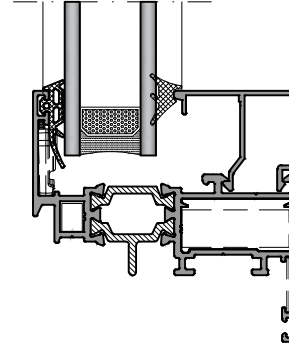
CAM KALINLIĞINA GÖRE CAM ÇİTASI SEÇİM TABLOSU KANAT-KANAT İÇİ ORTAKAYIT-ETEK PROFİLİ Glazing Bead Selection Table according to the Glass Thickness SASH-SASH MULION-BOTTOM RAIL PRO.
