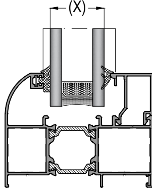
OVAL+ SERİ KASA CAM LİSTESİ
