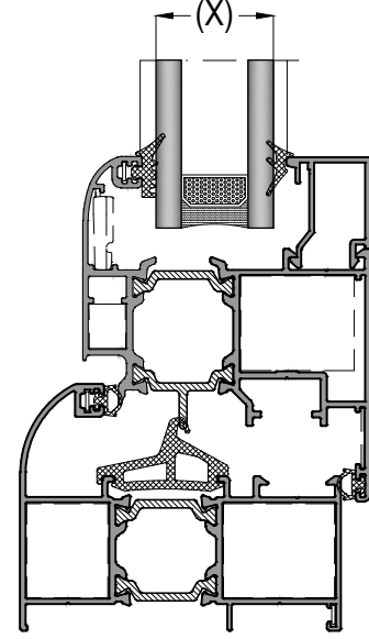
OVAL+ SERİ KANAT CAM LİSTESİ
