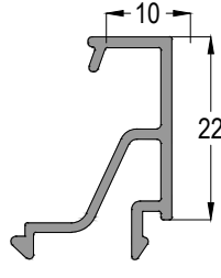
CAM KALINLIĞINA GÖRE CAM ÇİTASI SEÇİM TABLOSU Glazing Bead Selection Table according to the Glass Thickness (LS70-11)
