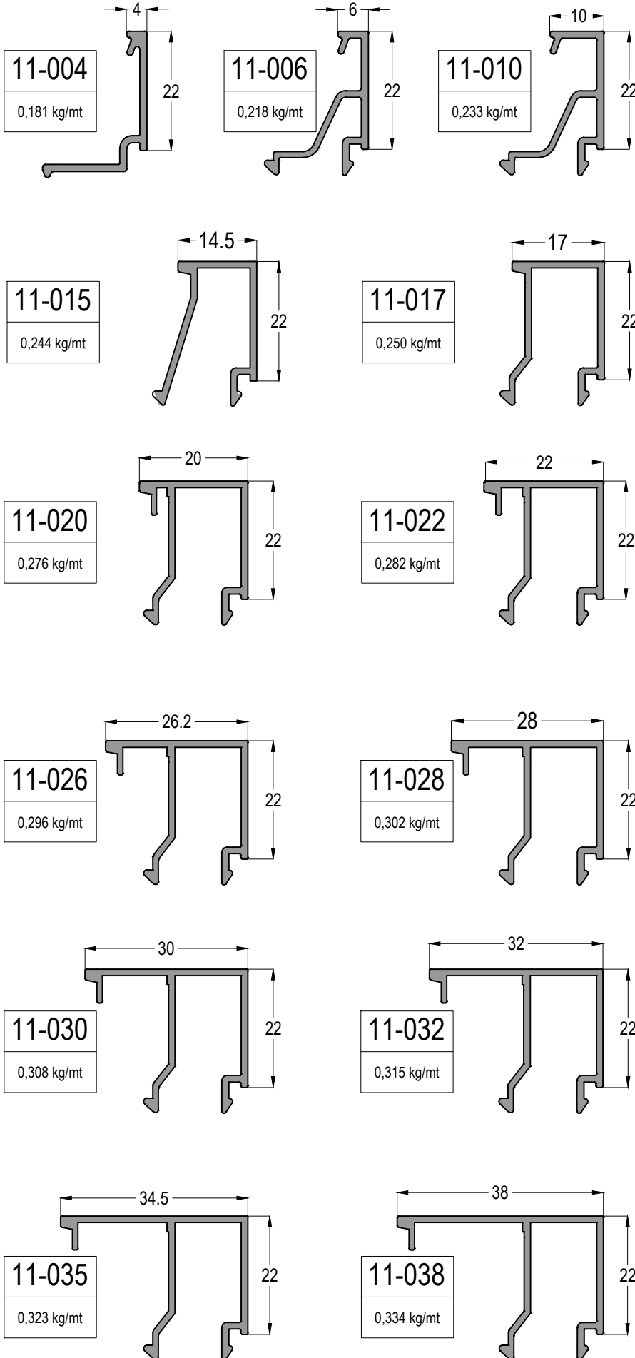
CAM KALINLIĞINA GÖRE CAM ÇITASI SEÇİM TABLOSU Glazing Bead Selection Table according to the Glass Thickness
