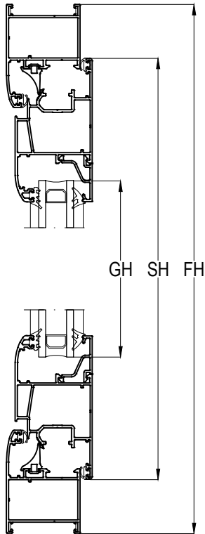
ADAPTÖR PROFİLİ AS42 42 = SH - 66mm
